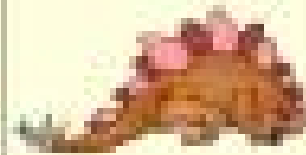
Stegosaurus
