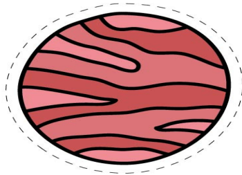
Venus
