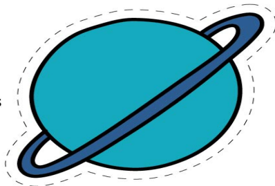
Uranus
