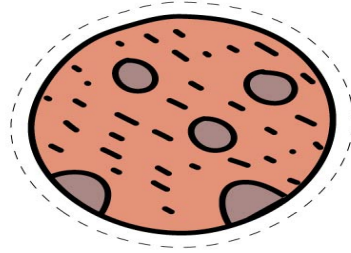
Mars
