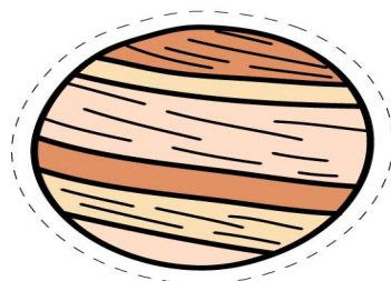
Jupiter
