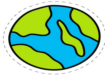
Earth
