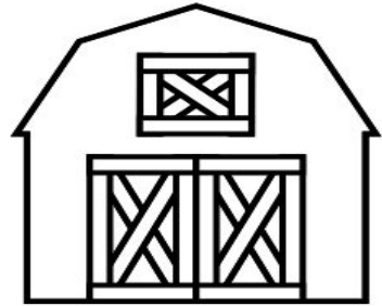
barn
